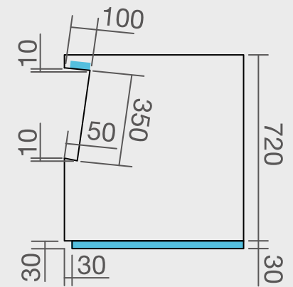
剖面图
